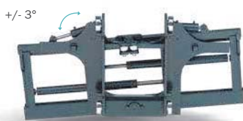
Piastra regolabile con livellamento (2 forche) per merci sensibili
