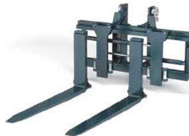
Piastra con fork shaft system (multifunzione), versione pin-type e hook-type
